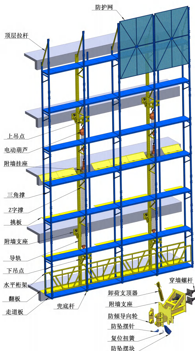
架体整体示意图
